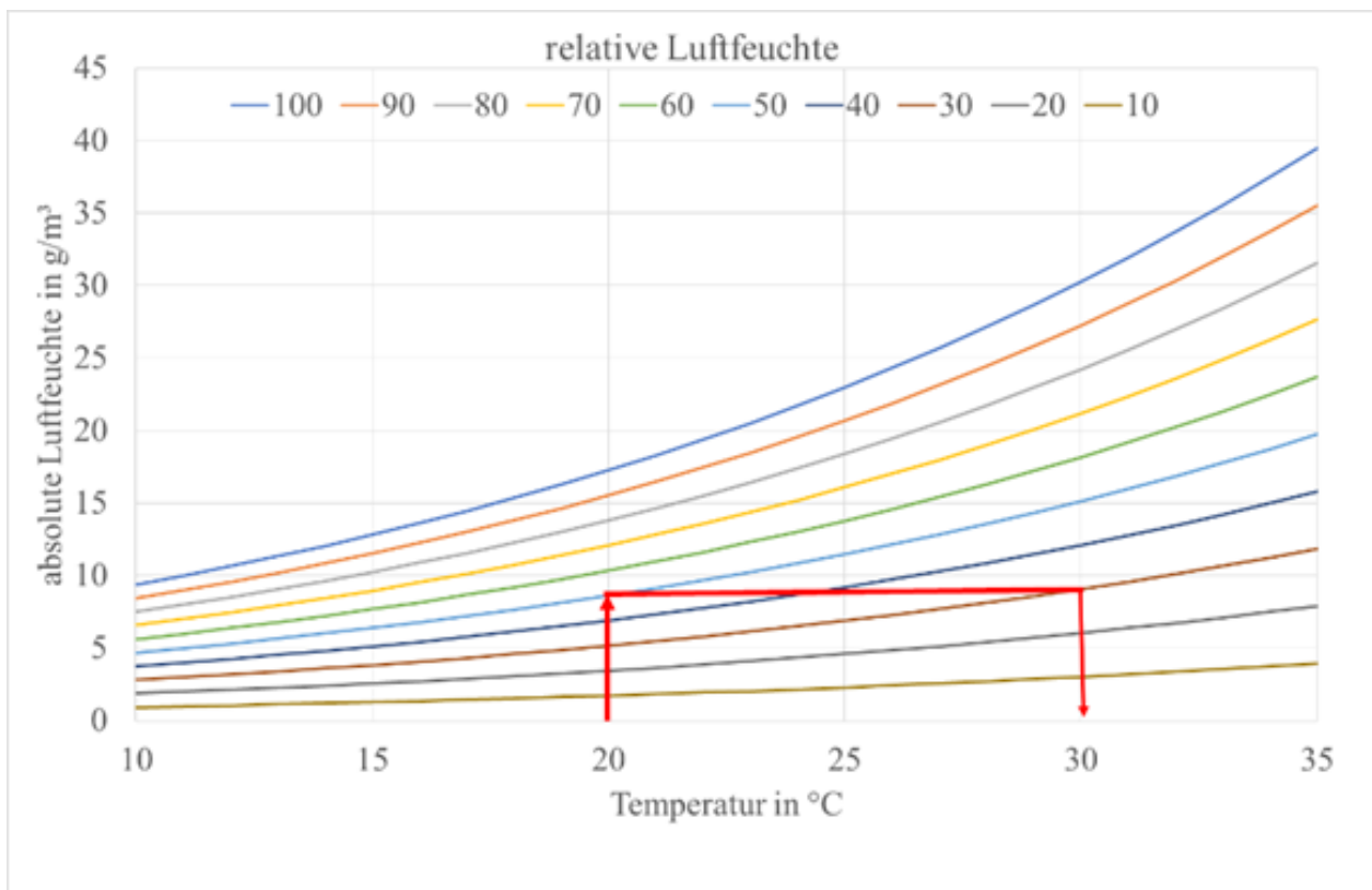
Diagramm 1: Relative Luftfeuchte in Abhängigkeit der absoluten Luftfeuchte und Temperatur.
